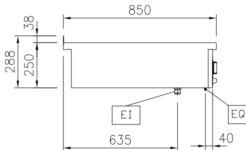
Zij aanzicht
